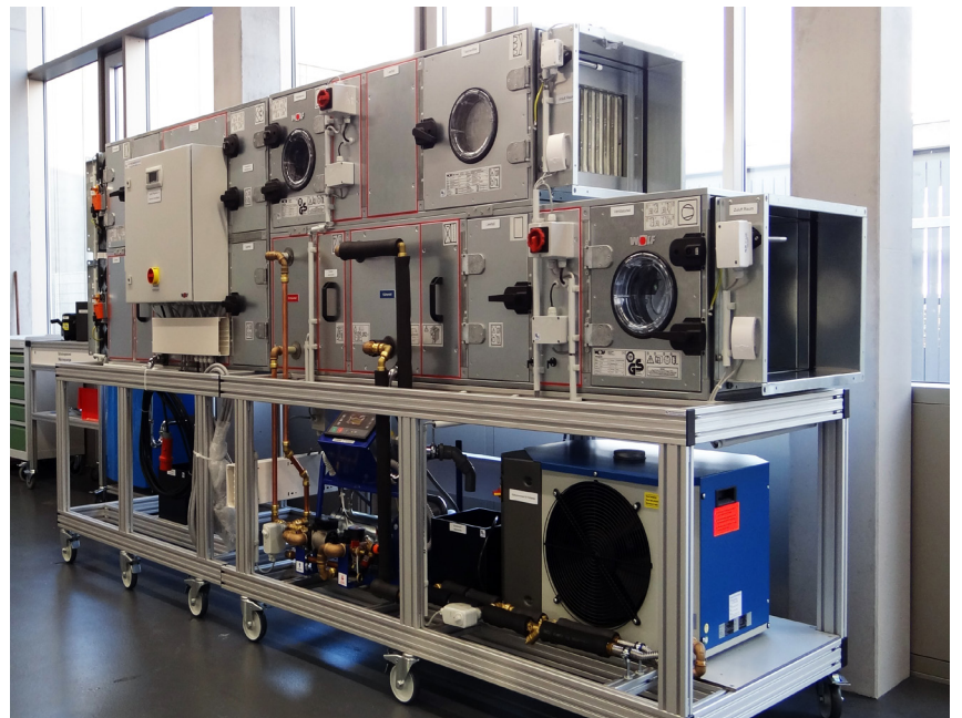
Schulungsstand Klimaanlage, Praxisausführung
